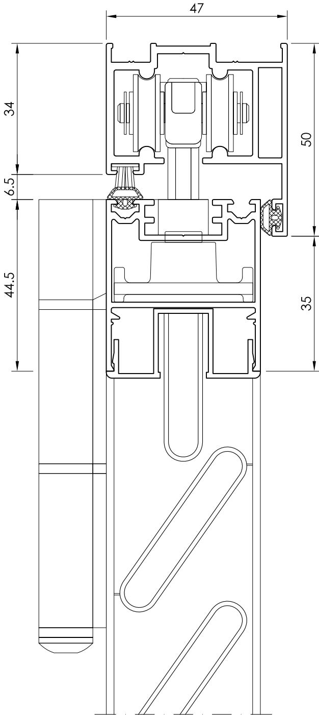
◀ Nudo Superior con guía de carros PI 65008
